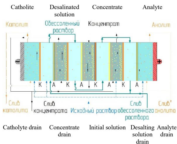
Рисунок 2. Схема электродиализного аппарата
