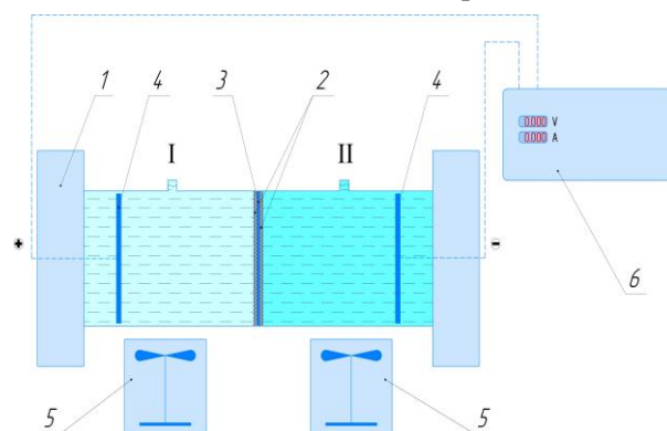
Рисунок 3. Экспериментальная электродиффузионная установка: 1 – прижимная плита; 2 – зажимная решетка; 3 – мембрана; 4 – электрод; 5 – магнитная мешалка; 6 – лабораторный источник питания
