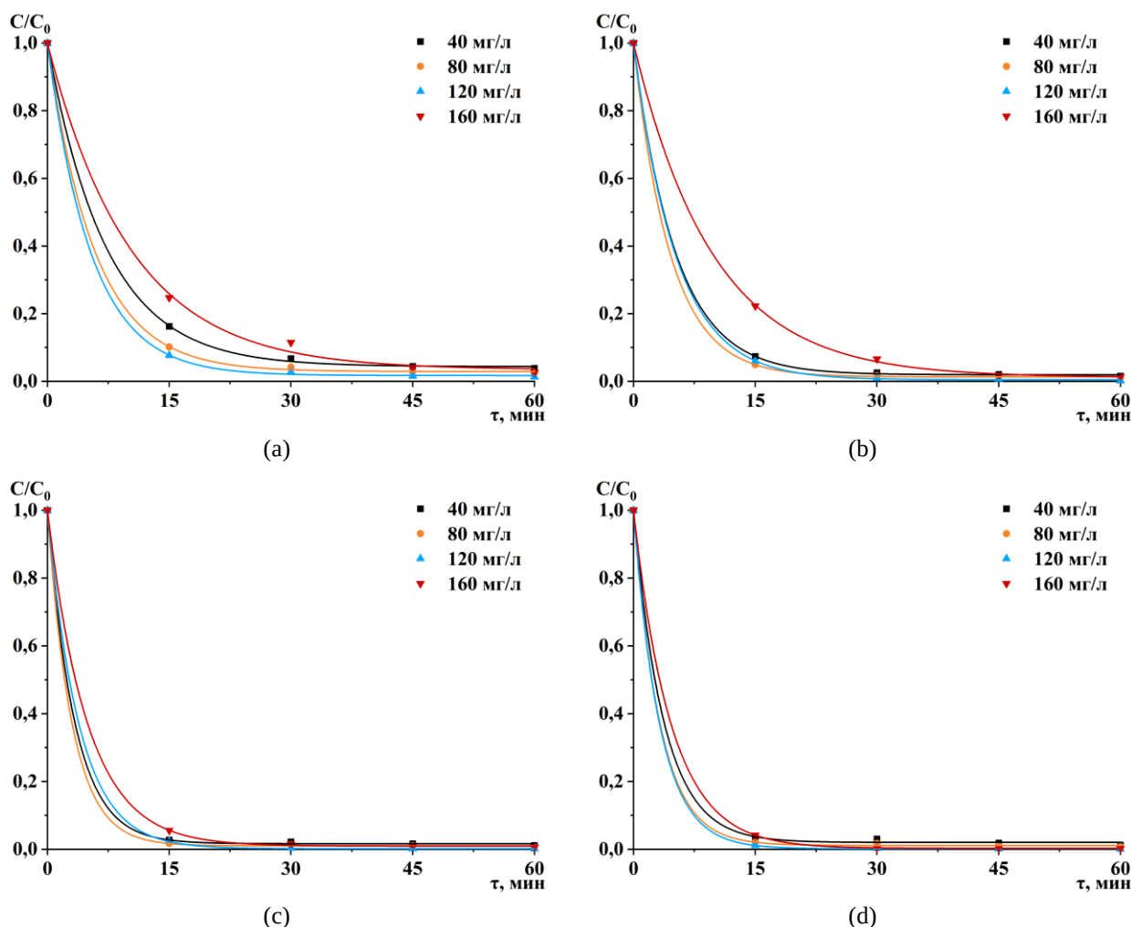
Рисунок 4. Кинетические зависимости концентрации C ионов Ni^{2+} , нормированной к исходной величине C_0 , от времени: (a) – 10 А/м 2 ; (b) – 20; (c) – 30 А/м 2 ; (d) – 40 А/м 2
