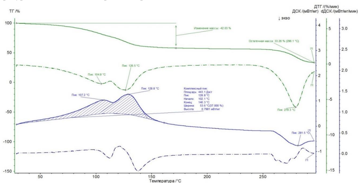
Рисунок 1. Термограмма образца хлеба без муки без обработки ТВС (контроль)
