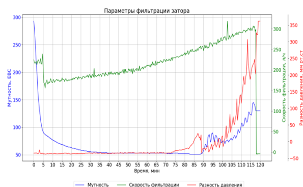
Рисунок 2. График фильтрации
