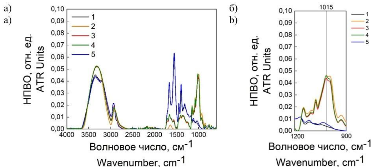
Рисунок 2. ИК-спектры (а) и фрагмент ИК-спектров в диапазоне 900–1200 см -1 , иллюстрирующий изменение интенсивности полосы 1015 см -1 (б): 1 – контрольный образец акрилового гидрогеля; 2 – биофунгицид «Триходермин»; 3 – акриловый гидрогель, модифицированный биофунгицидом «Триходермин» по схеме 1; 4 – акриловый гидрогель, модифицированный биофунгицидом «Триходермин» по схеме 2; 5 – акриловый гидрогель, модифицированный биофунгицидом «Триходермин» по схеме 3.
