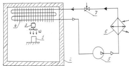
Рисунок 1. Схема холодильной камеры
