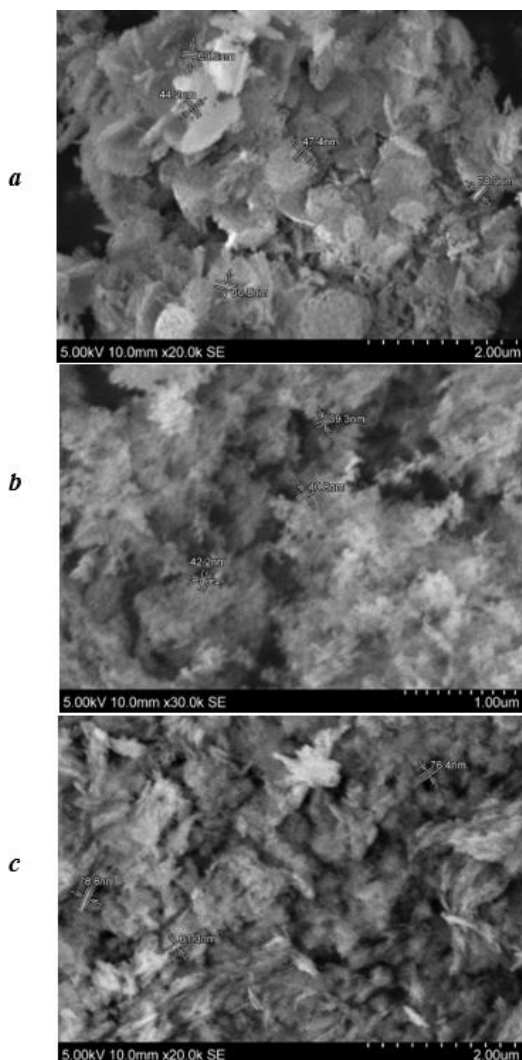
Рисунок. 3 Микрографии образцов оксида магния, полученных при помощи различных осадителей: а – осадитель \text{NH}_4\text{OH} , б – осадитель NaOH, с – осадитель \text{Ca}(\text{OH})_2
