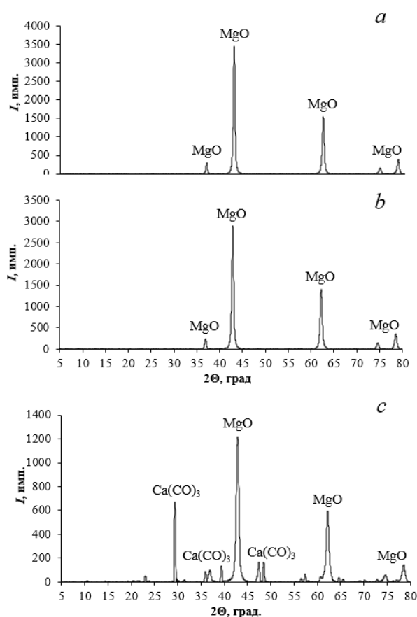
Рисунок. 2 Дифрактограммы образцов: а – \text{MgO-NH}_4\text{OH} ; б – \text{MgO-NaOH} ; в – \text{MgO-Ca}(\text{OH})_2
