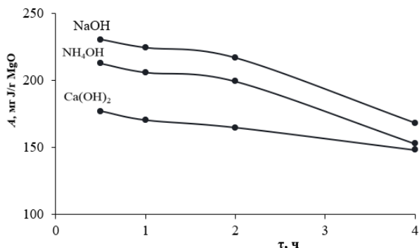
Рисунок. 4 Зависимость активности MgO от длительности прокаливания Mg(OH) 2
