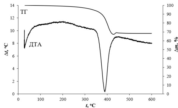
Рисунок. 1 Дериватограмма процесса дегидратации Mg(OH)_2
