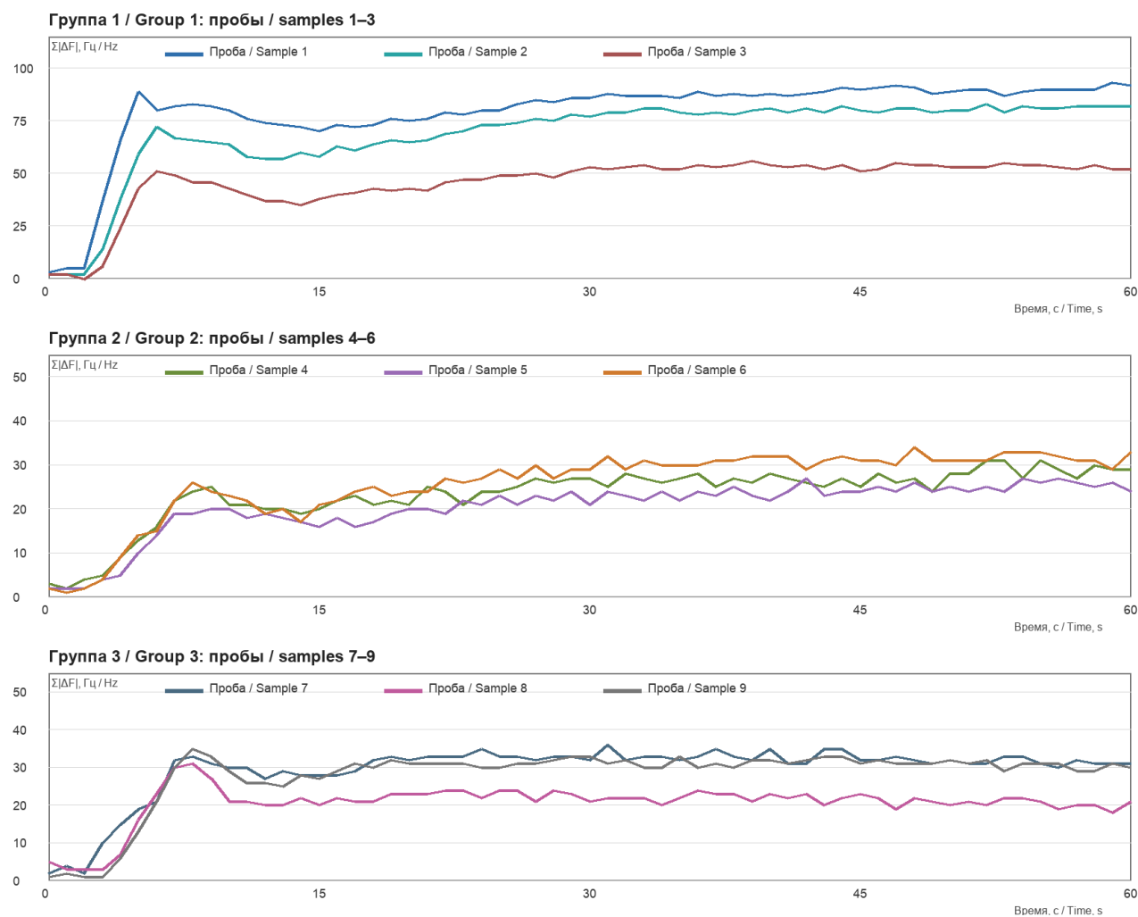
Рисунок 1. Динамика суммы модулей откликов восьми сенсоров за 60 с Figure 1. Dynamics of the summed absolute responses of eight sensors over 60 s
