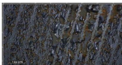
Рисунок 4. Разрушение лакокрасочного покрытия и коррозия после стерилизации в 3% растворе пищевой соли Figure 4. Destruction of paint coating and corrosion after sterilization in 3% solution of edible salt
