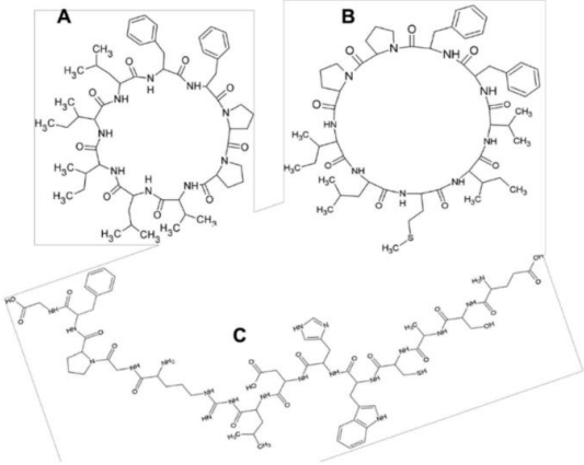
Рисунок 8. Химические структуры пептидов белка льняного семени: (А) Циклолинопептид-А; (В) Циклолинопептид-В; (С) антиоксидантный пептид, полученный, гидролизом белка алкалазой [19]
