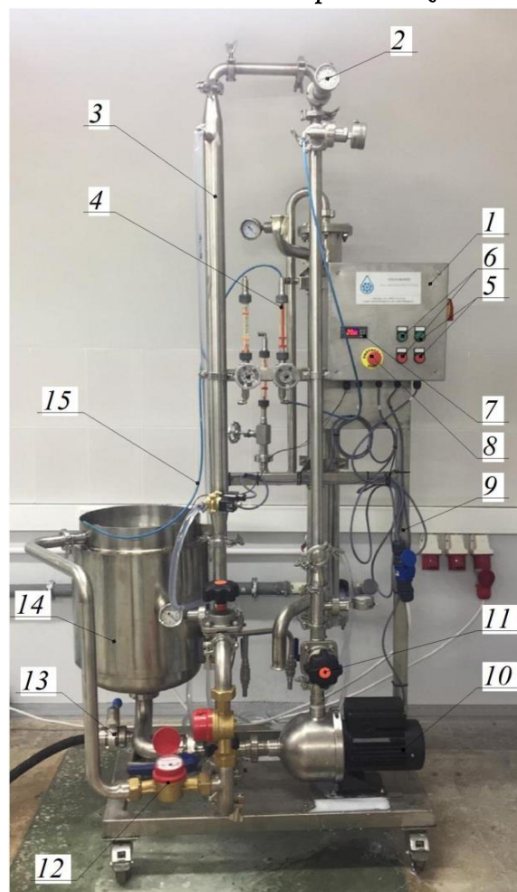
Рисунок 1. Баромембранная установка: 1 – щит управления, 2 – манометр, 3 – теплообменник, 4 – ротаметр, 5 – кнопки пуск/стоп электродвигателя, 6 – кнопки контроля датчика температуры, 7 – датчик контроля температуры, 8 – кнопка отключения установки, 9 – рама, 10 – насос, 11 – задвижка, 12 – расходомер, 13 – кран для слива концентрата, 14 – емкость, 15 – трубка для слива пермеата
