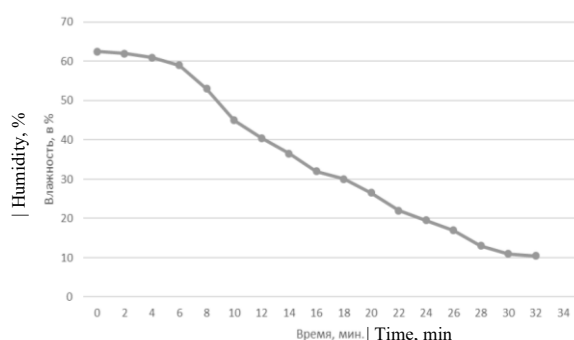
Рисунок 2. Динамика изменения влажности рафината в процессе сушки при мощности СВЧ 540 Вт
