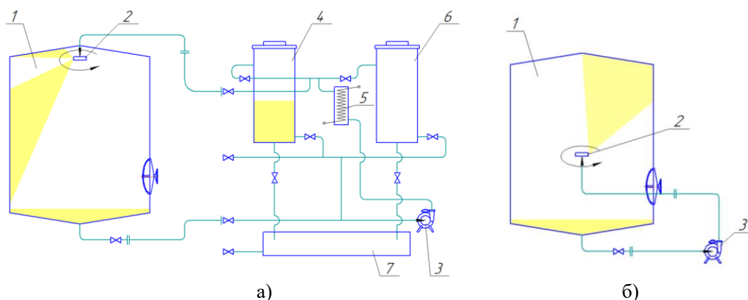
Рисунок 1. Схемы мойки технологического оборудования пивоварни: а) с использованием передвижной CIP-станции; б) в циркуляционном режиме: 1 – емкость; 2 – вращающаяся форсунка; 3 – насос; 4 – емкость оборотного моющего щелочного раствора; 5 – электрический нагреватель проточного типа; 6 – емкость оборотного дезинфицирующего раствора (не используется); 7 – емкость для нейтрализации щелочного раствора.
