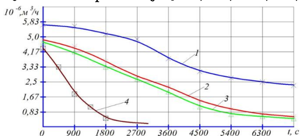
Рисунок 2. Зависимости производительности баромембранной установки (по фильтрату) от времени t , с
