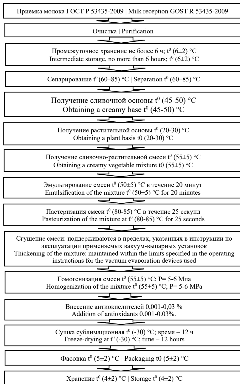
Рисунок 1. Технологическая схема 1 процесса производства сухого сливочно-растительного спреда.
