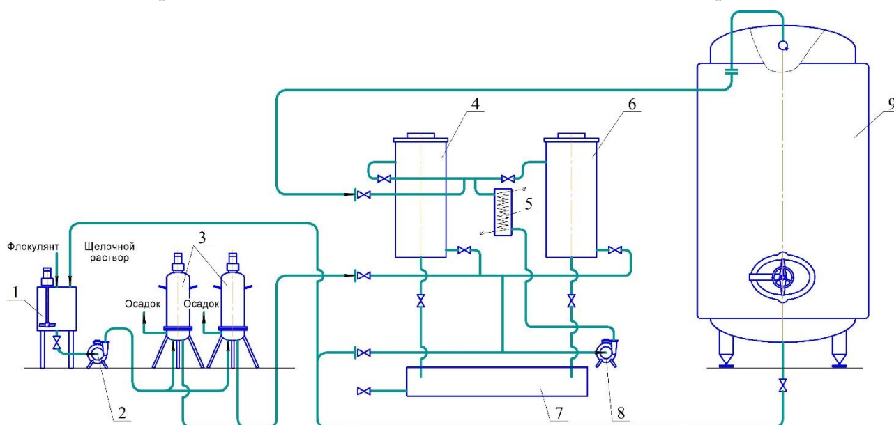
Рисунок 9. Схема регенерации моющего щелочного раствора с использованием флокулянтов: 1 – смеситель; 2 – центробежный насос; 3 – самопромывной фильтр; 4 – емкость оборотного моющего щелочного раствора; 5 – электрический нагреватель проточного типа; 6 – емкость оборотного дезинфицирующего раствора (не используется); 7 – емкость для нейтрализации щелочного раствора; 8 – циркуляционный насос; 9 – емкость для мойки и дезинфекции
