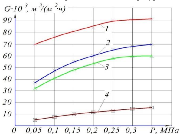
Рисунок 3. Зависимости проницаемости УФ мембран от давления (по фильтрату при T = 293 K)
