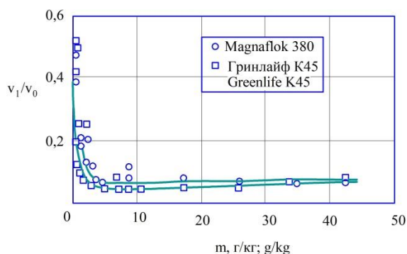
Рисунок 4. Влияние количества флокулянта, m , г/кг на соотношение скоростей витания и осаждения v_1/v_0 примесей в моющем щелочном растворе
