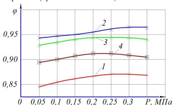
Рисунок 4. Зависимости селективности УФ мембран от давления (по фильтрату при T = 293 K)
