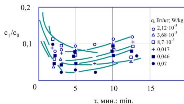
Рисунок 6. Влияние изменения величины удельных затрат энергии q , Вт/кг и продолжительности перемешивания на соотношение содержания твердых веществ в осветленном растворе к содержанию твердых веществ в исходном моющем щелочном растворе c_1/c_0 .
