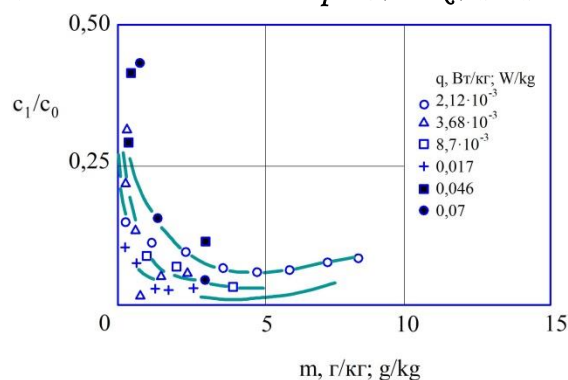
Рисунок 5. Влияние изменения величины удельных затрат энергии q , Вт/кг и количества, вносимого флокулянта на соотношения содержания твердых веществ в осветленном растворе к содержанию твердых веществ в исходном моющем щелочном растворе c_1/c_0 .
