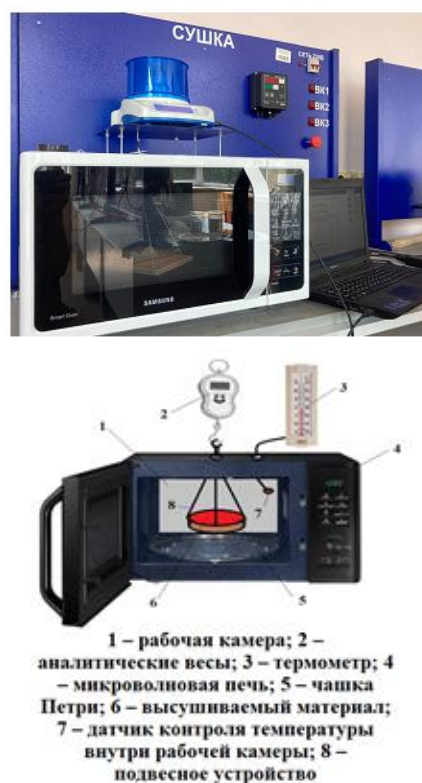
Рисунок 1. – Лабораторный стенд для определения кинетических показателей процесса сушки»
