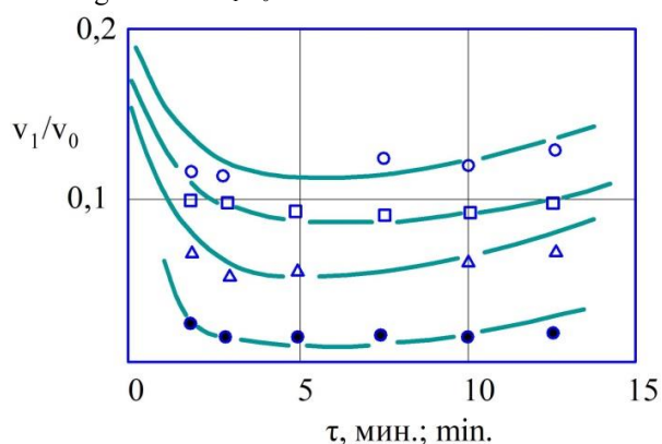
Рисунок 8. Влияние продолжительности обработки \tau , мин на соотношение скоростей витания и осаждения v_1/v_0 примесей в моющем щелочном растворе, при различных значениях затрат энергии (обозначения кривых, соответствуют рисунку 6).
