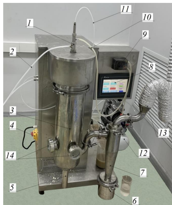
Рисунок 5. Распылительная сушилка УС-500: 1 – форсунка, 2 – трубка подачи сжатого воздуха, сушильная камера, 4 – тумблер питания, 5 – сборник конденсата, 6 – приемная емкость, 7 – циклонный сепаратор, 8 – панель управления, 9 – перистальтический насос, 10 – трубка подачи продукта, 11 – трубка защиты системы от засорения, 12 – компрессор, 13 – отвод отработанного воздуха, 14 – смотровое окно
