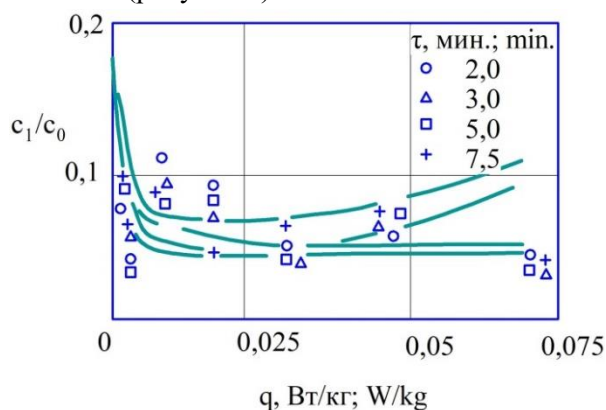
Рисунок 7. Влияние продолжительности перемешивания и изменения величины удельных затрат энергии q , Вт/кг на соотношения содержания твердых веществ в осветленном растворе к содержанию твердых веществ в исходном моющем щелочном растворе c_1/c_0 .
