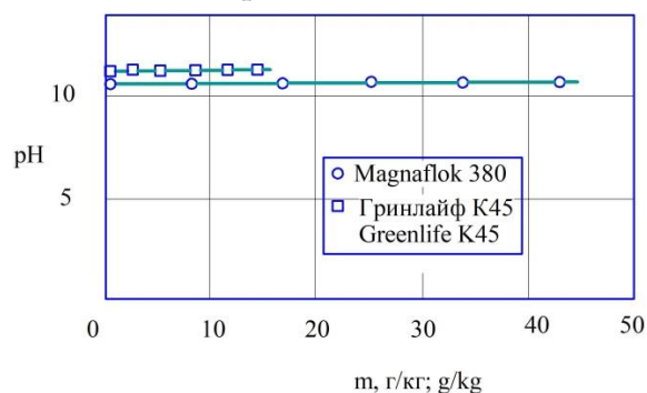
Рисунок 3. Влияние количества флокулянта, m , г/кг на величину активной кислотности pH моющего щелочного раствора
